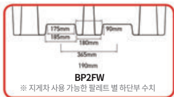
BP2FW 205리터 드럼 2개 보관에 적합 *4방향(4-way)으로 지게차 사용 가능
