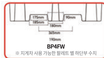
BP4FW 205리터 드럼 4개 보관에 적합 *4방향(4-way)으로 지게차 사용 가능
