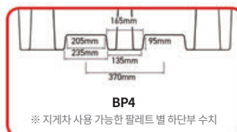
BP4 205리터 드럼 4개 보관에 적합 *양방향 (2-way)으로 지게차 사용 가능
